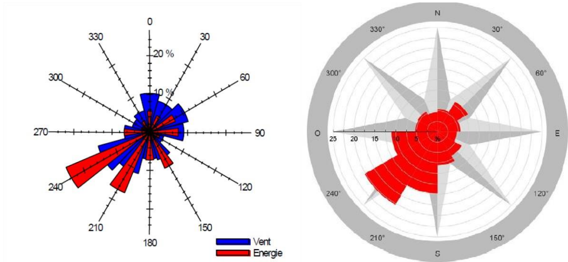
Rose des vents (à gauche) et rose des vents énergétique (à droite) sur le site d'implantation – TotalEnergies
