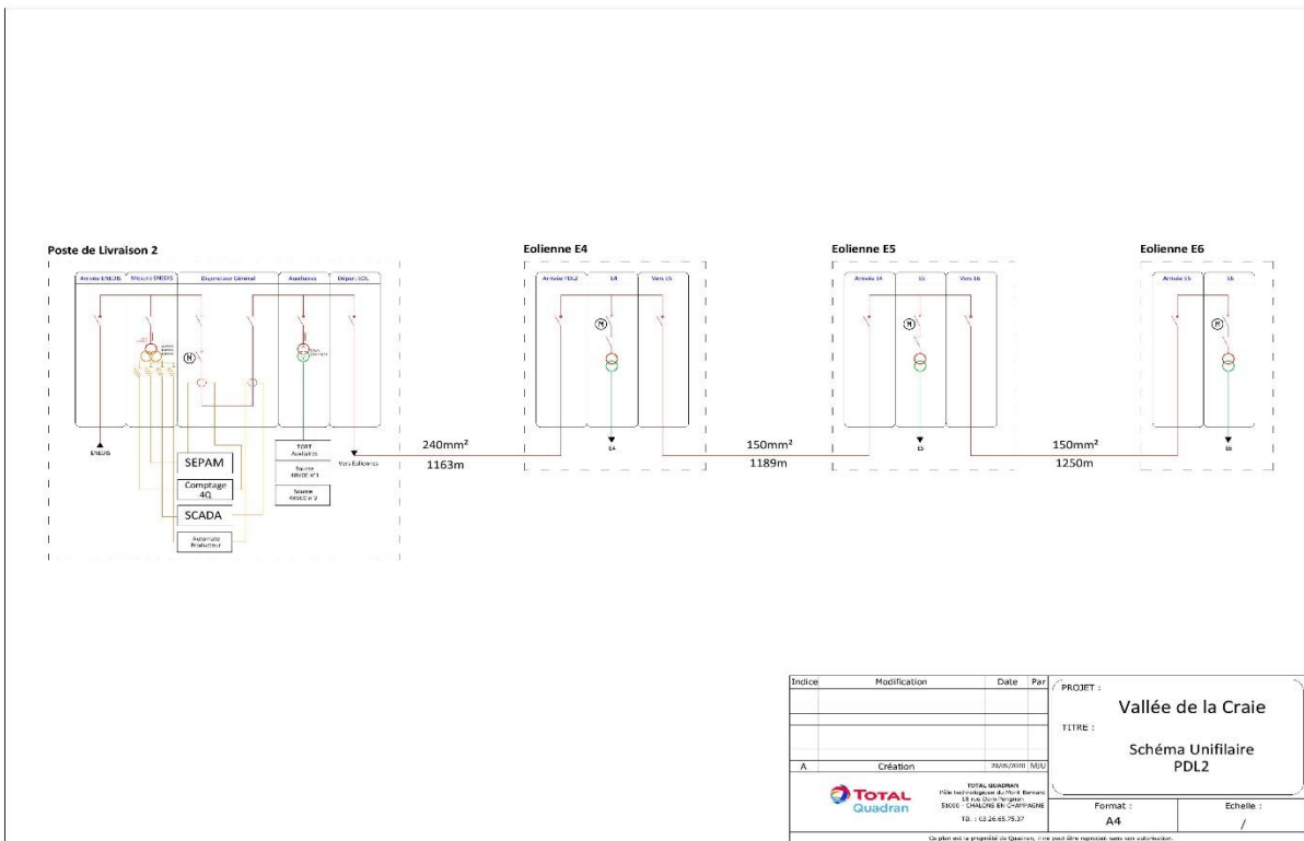
Schéma unifilaire du poste de livraison 2
