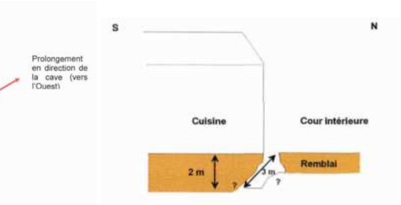
Coupe S-N de l'extension de la cavité
