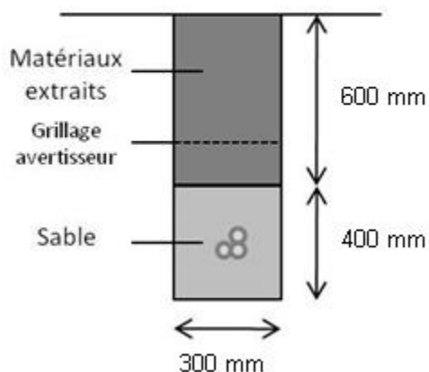
Coupes générales des tranchées destinées à l'enfouissement des lignes électriques
