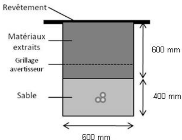
Coupes générales des tranchées destinées à l'enfouissement des lignes électriques
