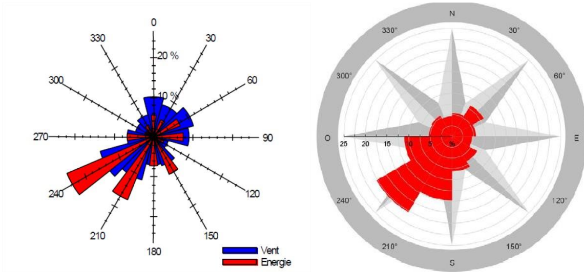
Rose des vents (à gauche) et rose des vents énergétique (à droite) sur le secteur d'étude – TOTALENERGIES
