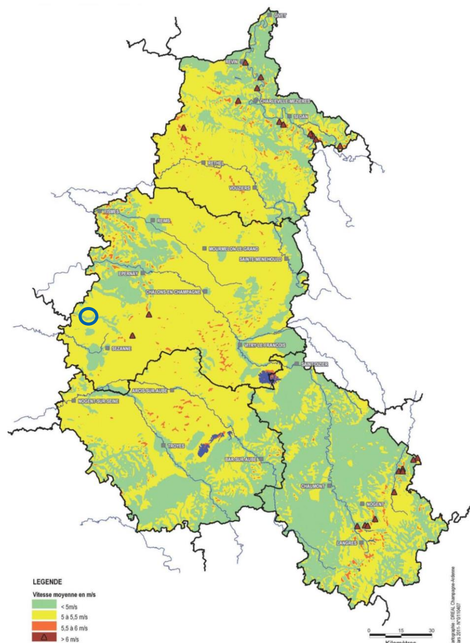
Carte 6 : Vitesse des vents dans l'ancienne région Champagne-Ardenne – Cercle bleu : Périmètre d'étude de dangers (source : Schéma Régional Eolien, 2012)
