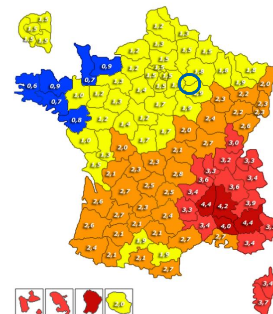
Carte 10 : Densité de foudroiement – Cercle bleu : Périmètre d'étude de dangers (source : Météo Paris, 2021)
