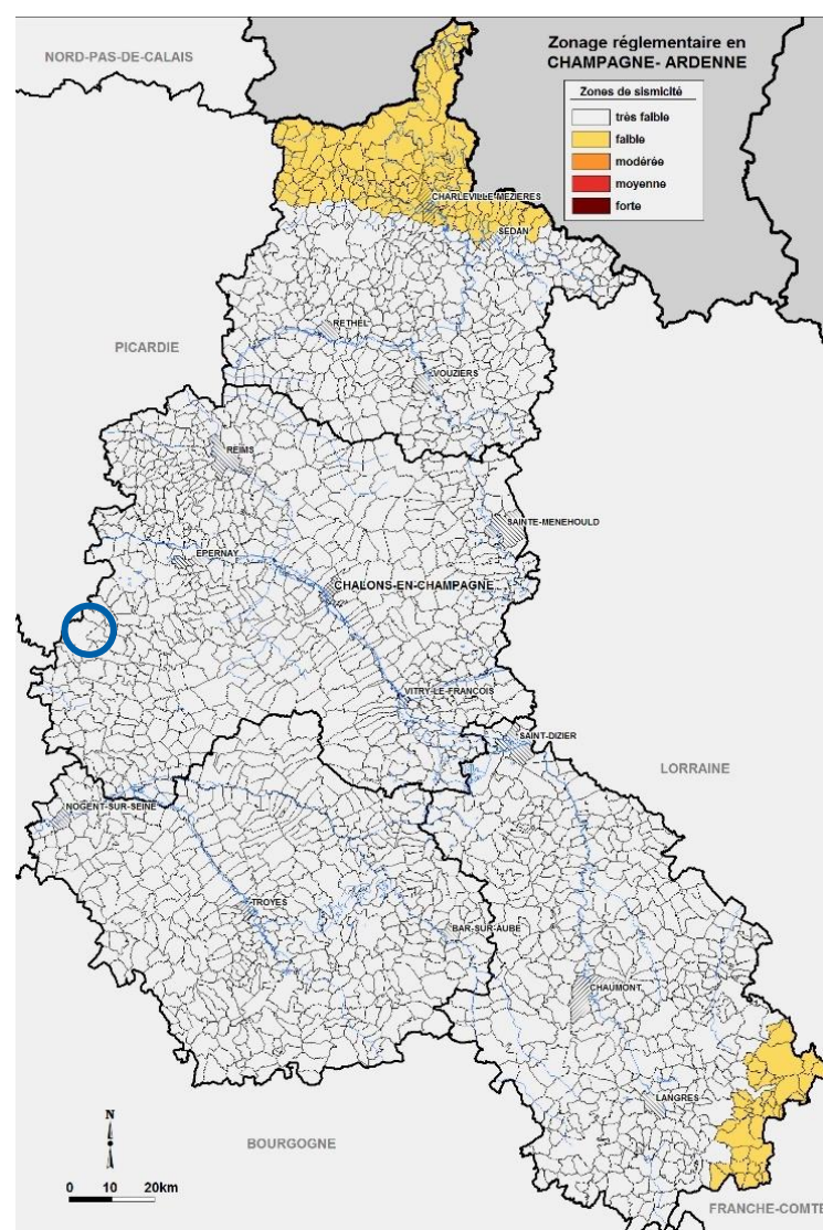
Carte 9 : Zonage sismique de l'ancienne région Champagne-Ardenne – Cercle bleu : zone d'implantation potentielle (source : planseisme.fr, 2015)
