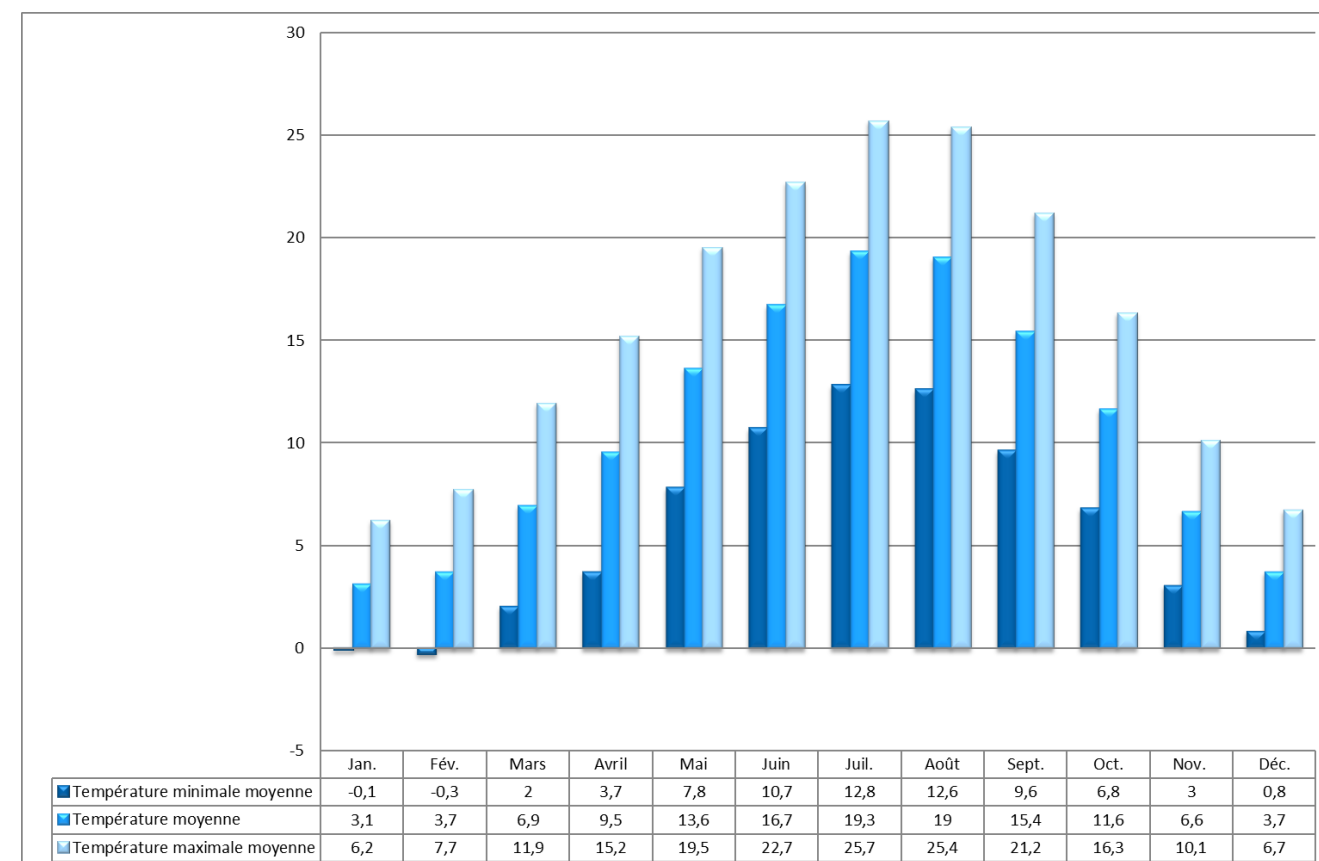
Figure 3 : Illustration des températures de 1981 à 2010 – Station de Troyes-Barbery (source : Infoclimat.fr, 2019)
