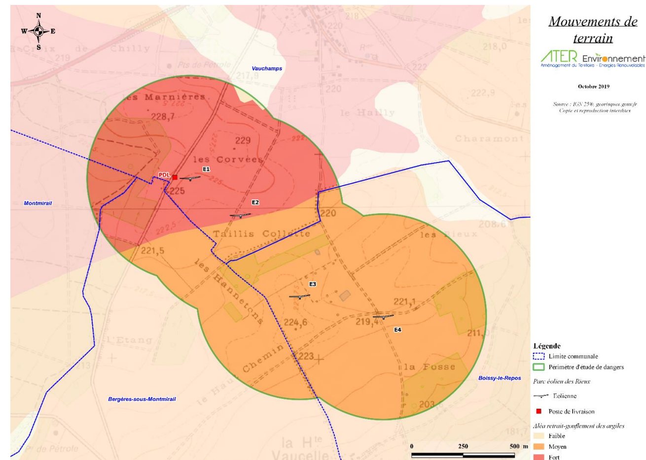
Carte 8 : Aléa retrait-gonflement des argiles (source : www.argiles.fr , 2021)
