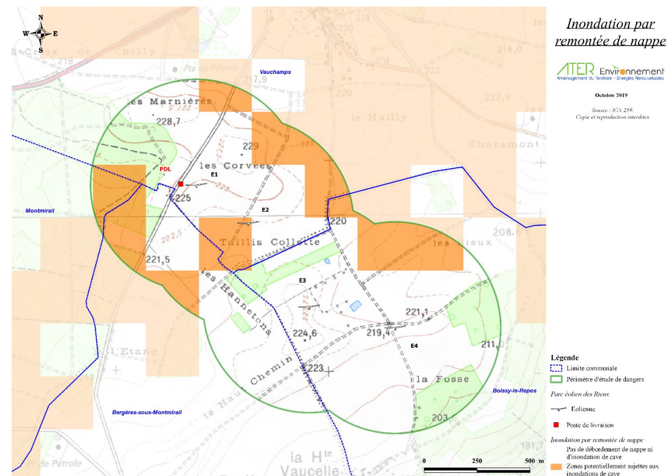
Carte 7 : Sensibilité du périmètre d'étude de dangers au phénomène d'inondation par remontée de nappe (source : georisques.gouv.fr)
