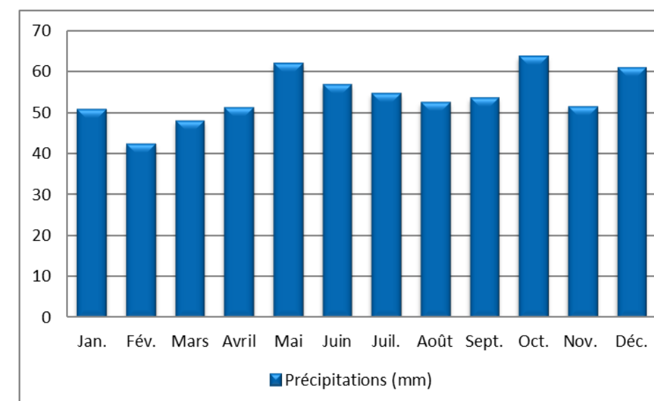
Figure 4 : Illustration des précipitations de 1981 à 2010 – Station de Troyes-Barbery (source : Infoclimat, 2019)
