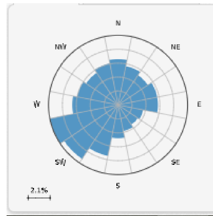
Figure 5 : Rose des vents (source : VALECO, 2019)
