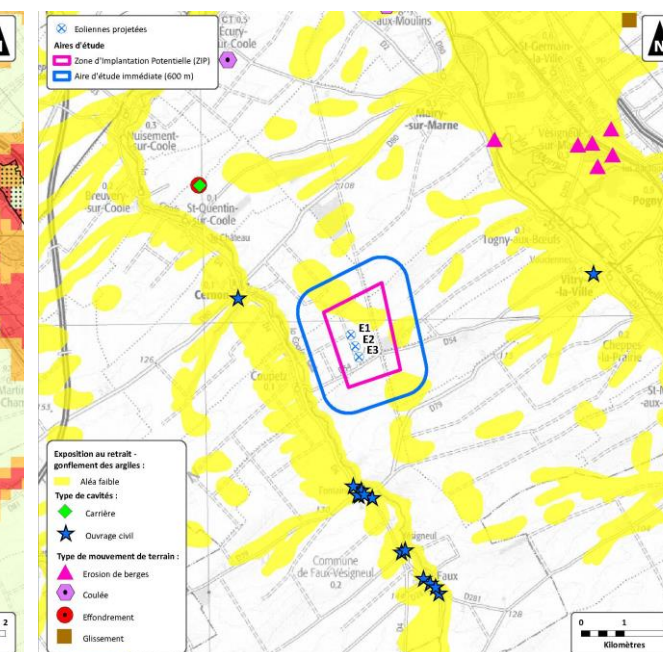
Carte 4. Risques naturels (mouvements de terrain, argiles, cavités)
